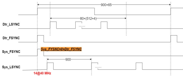
图6 探测器驱动时序图
