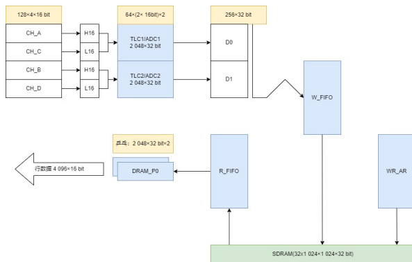
图11 数据采集和控制框图 Fig. 11 Data acquisition and control block diagram
