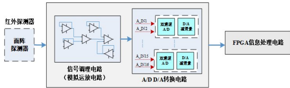
图5 前端信号调理图
