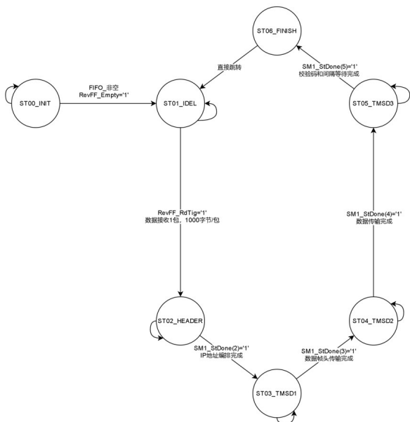
图10 数据传输状态机 Fig. 10 Data transmission state machine
