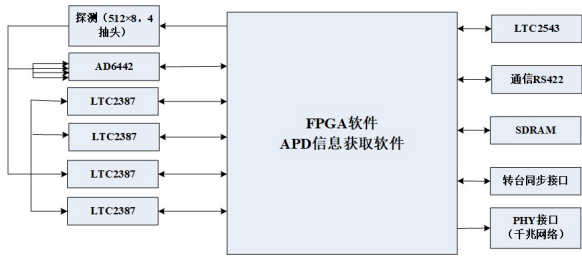
图4 红外信息获取系统框图
