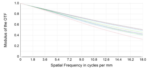
图3 光学系统传递函数图
