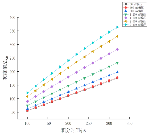
图 16 不同积分时间不同偏压下的黑体响应 Fig. 16 Blackbody response under different integration times and different bias
